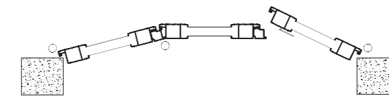
TP-LIB Persiana a tre ante pieghevoli
