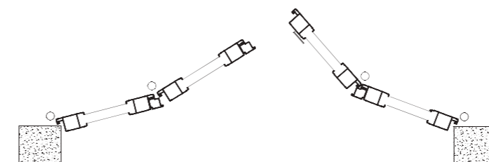
CP Persiana a quattro ante pieghevoli
