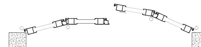
CP-LIB Persiana a quattro ante pieghevoli
