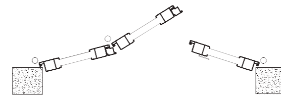
TP Persiana a tre ante pieghevoli
