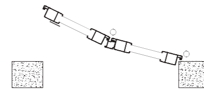
DP Persiana a due ante pieghevoli
